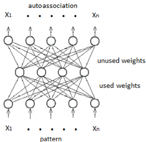
Autokodér na druhé nejnížší (první skryté) vrstvě DNN
