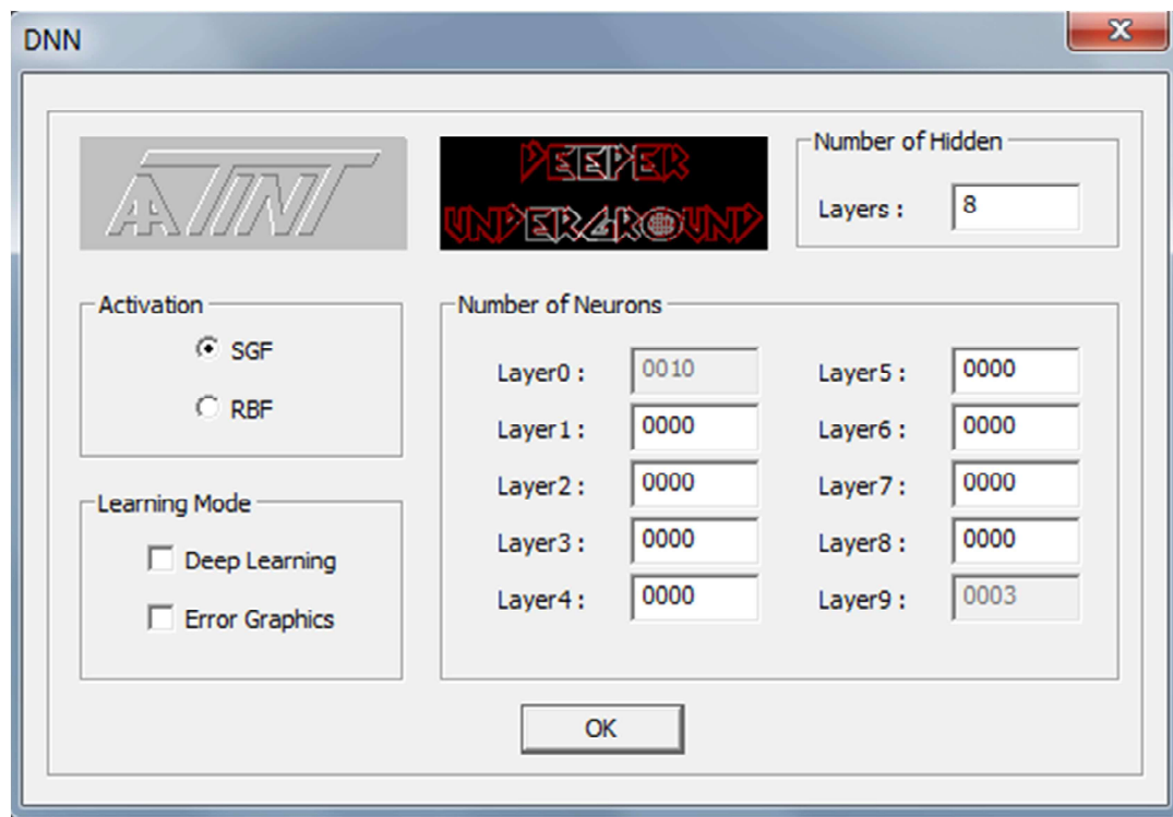
Parametrizace architektury DNN
